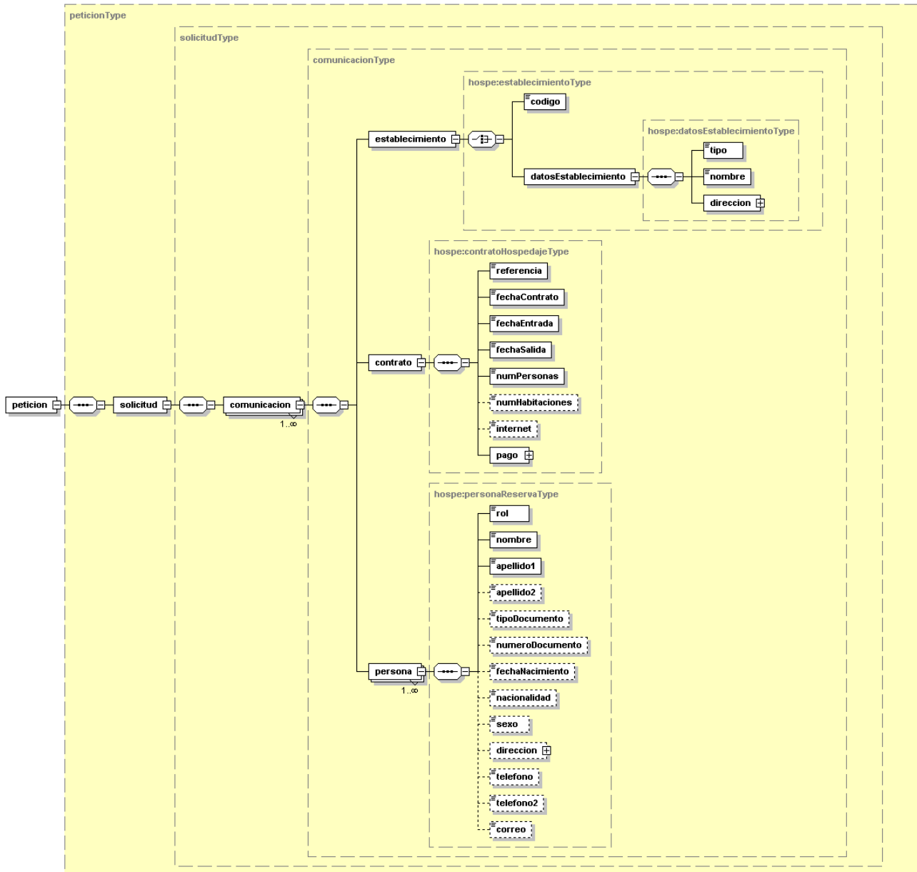
Figura 2. Plantilla para el alta de reservas de hospedaje
