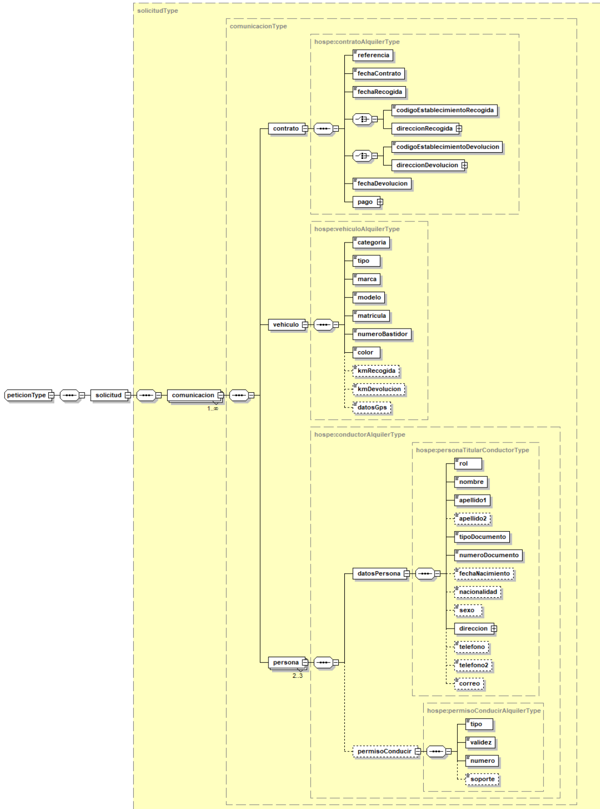
Figura 3. Plantilla para el alta de alquileres de vehículos
