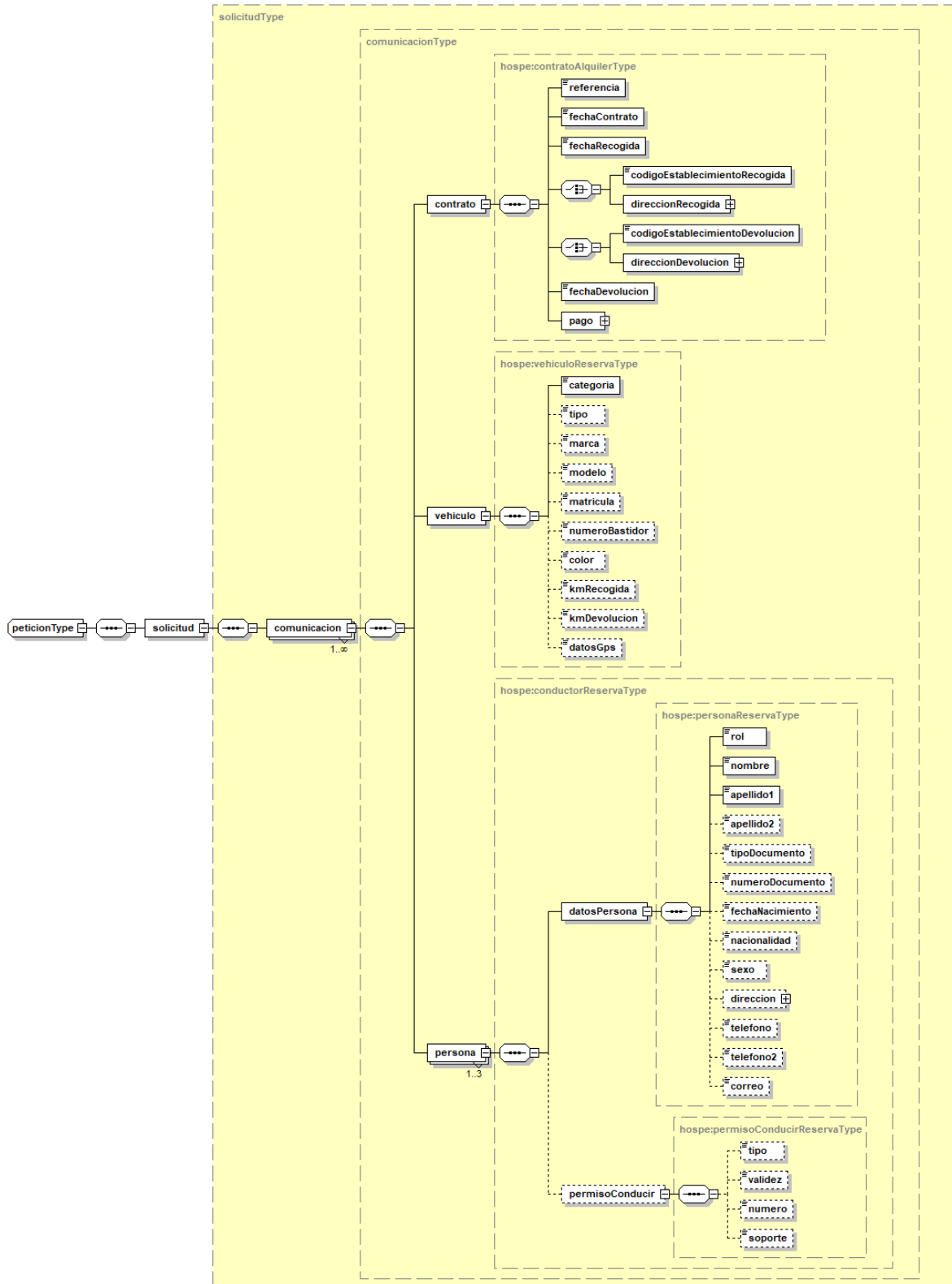
Figura 4. Plantilla para el alta de reservas de vehículos de alquiler
