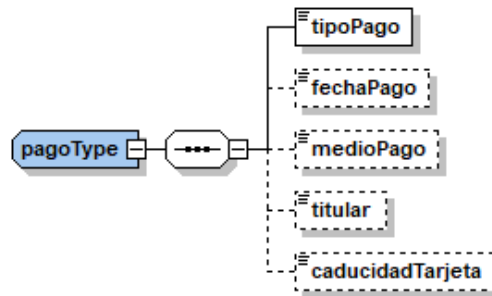
Figura 6. Bloque común pago
