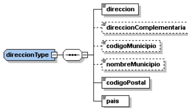
Figura 5. Bloque común direccion
