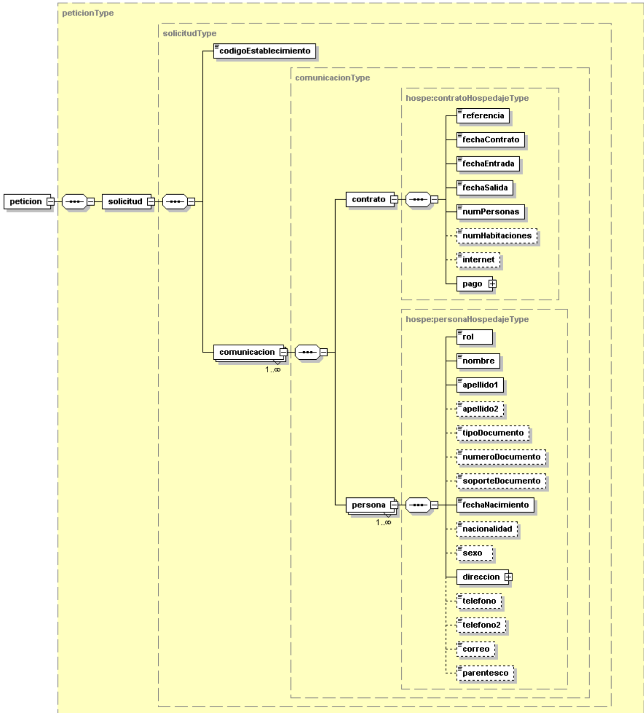
Figura 1. Plantilla para el alta de partes de viajeros
